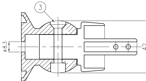
A-A 断面図
