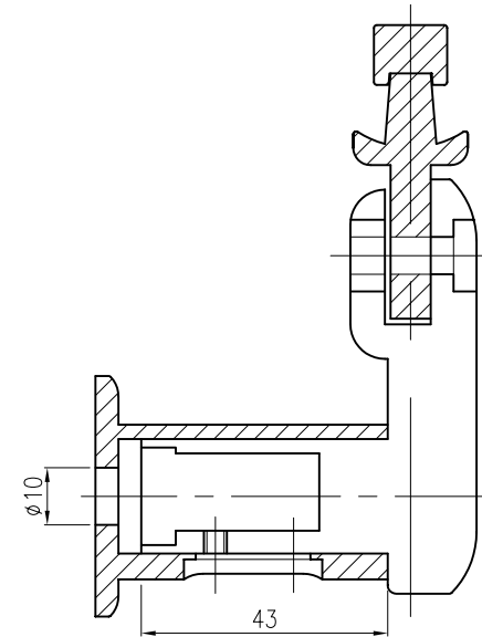
A-A 断面図
