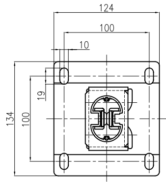
A-A断面図
