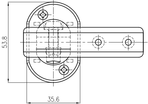
上面図 (S=1/1)
