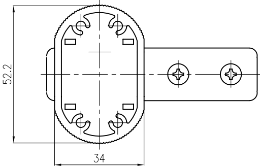
底面図 (S=1/1)
