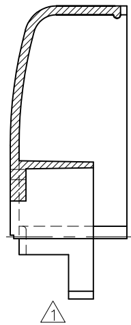
A-A 断面図
