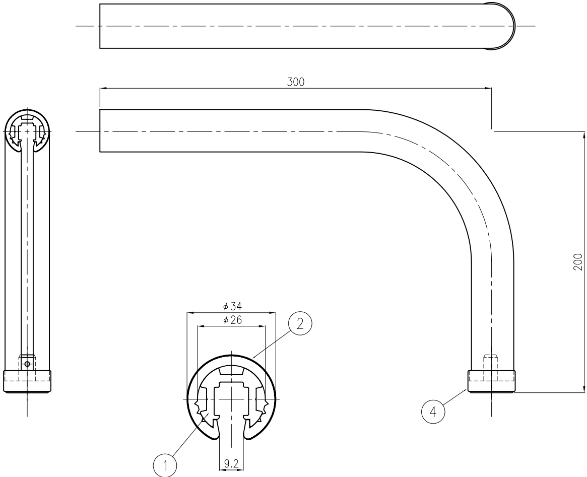
本体断面図 (S=1/1)
