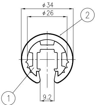
本体断面図 (S=1/1)
