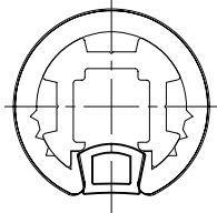
アンダーカバー 加合図 (S=1/1)
