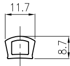
アンダーカバー断面図 (S=1/1)
